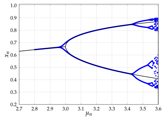
(b) Dynamique : \epsilon = -3 \cdot 10^{-4} .
