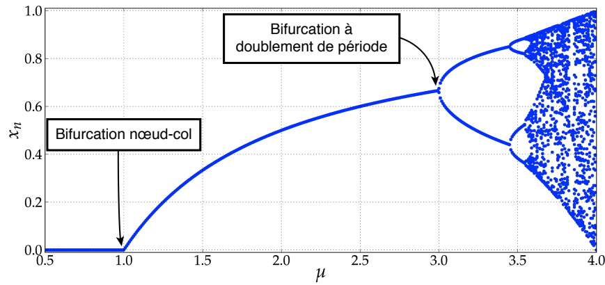
(a) Statique : \epsilon = 0 .
