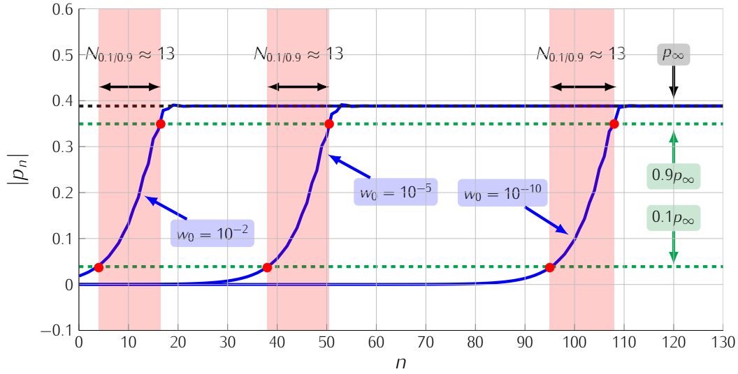
FIGURE 1.12 – Enveloppe temporelle de la pression p dans le bec reconstruite à partir de la variable x (solution de (1.33), ) en utilisant les équations (1.21) et (1.30). Le profil de l'onde aller x est obtenu pour w_0 = 10^{-2} , w_0 = 10^{-5} et w_0 = 10^{-10} . La longueur du transitoire N_{0.1/0.9} définie par l'équation (1.54) est indiquée pour chacune des trois enveloppes. \gamma = 0.42 , \zeta = 0.5 et \lambda = 1 .
