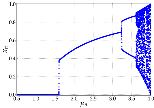
(b) Dynamique : \epsilon = 3 \cdot 10^{-4} .
