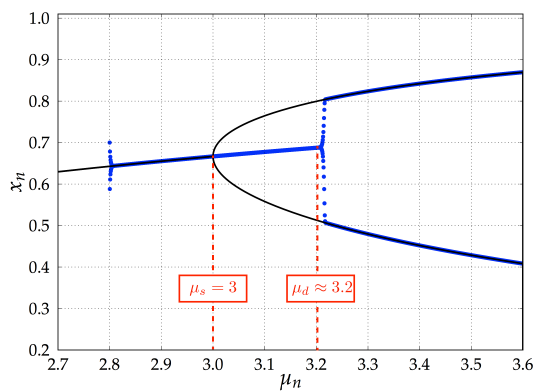
(a) Dynamique : \epsilon = 3 \cdot 10^{-4} .
