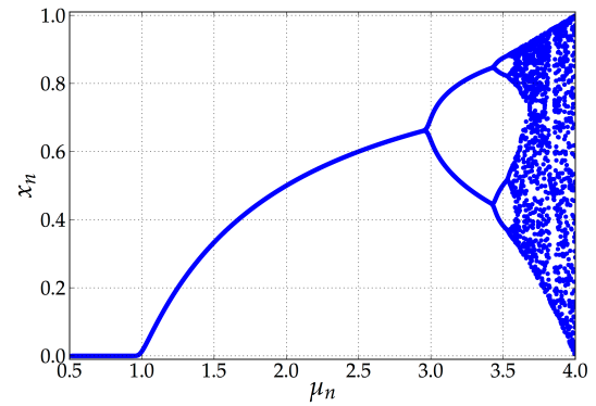
(c) Dynamique : \epsilon = -3 \cdot 10^{-4} .
