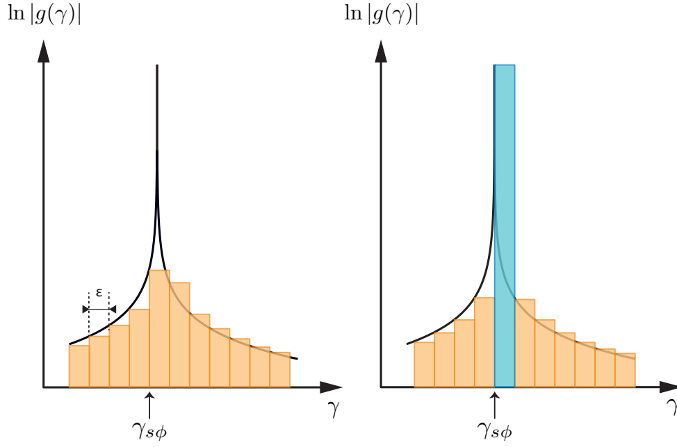
FIGURE C.3 – Comparaison entre la somme \epsilon \sum_{k=1}^n \ln |g(\gamma_k)| et l'intégrale \int_{\gamma_0+\epsilon}^{\gamma_0+\epsilon+\epsilon} \ln |g(\gamma')| d\gamma' . À gauche : aucune itération de \gamma_n n'est égale à \gamma_{s\phi} . À droite : l'une des itération de \gamma_n est égale à \gamma_{s\phi} .
