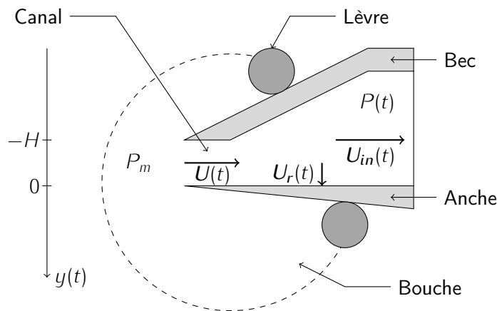
FIGURE 1.3 – Schéma de principe d'un bec à anche simple de type bec de clarinette ou de saxophone. Notations et orientations choisies.
